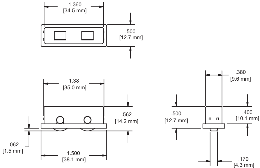
FIG. 2 4231-1000 ROLLER
